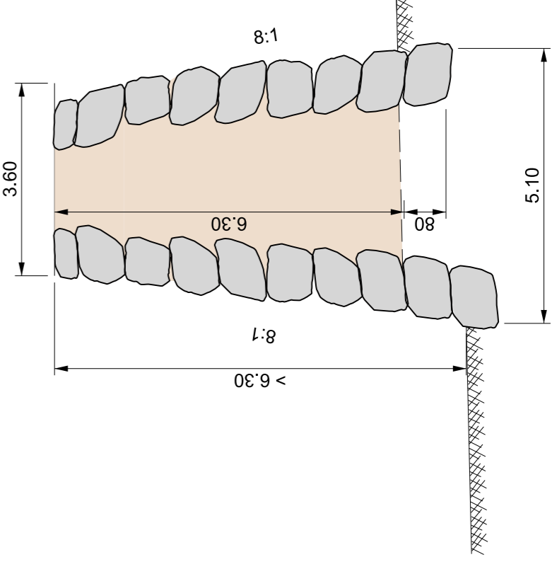
Profil B - B' 1:100
